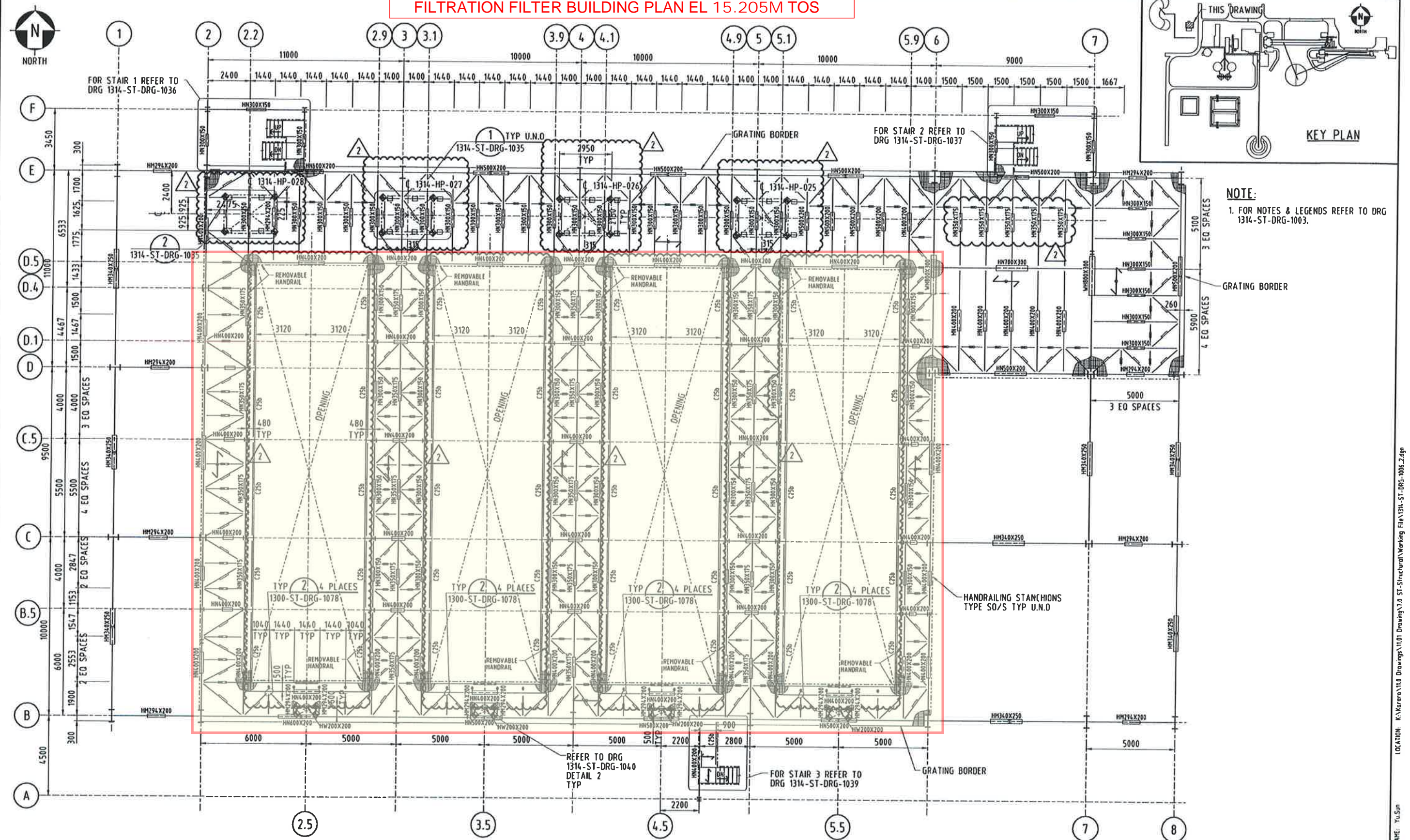
PLAN AT EL 15.205m TOS
